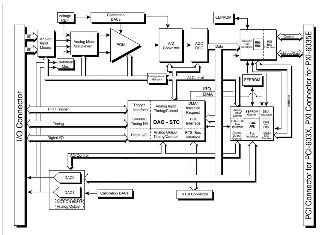
Figure 3-1. 6034E and 6035E Block Diagram
