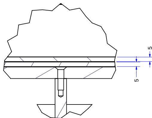
SECTION A-A SCALE 0.12 : 1
