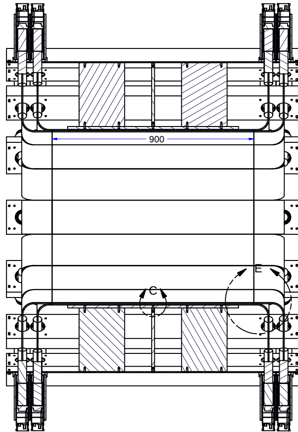
SECTION A-A SCALE 0.12 : 1
